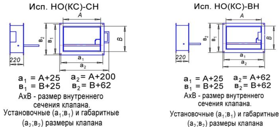
Рис. 1. Установочные, габаритные и размеры внутреннего сечения клапана.
